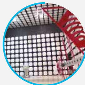
Cámara semianecoica de 10 m, marca ETS-Lindgren
